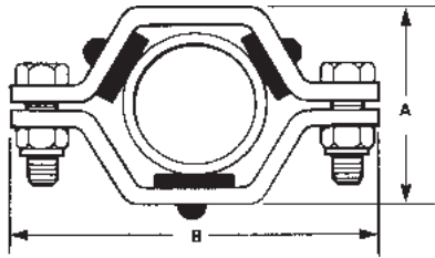
B24W Tubing Hanger
